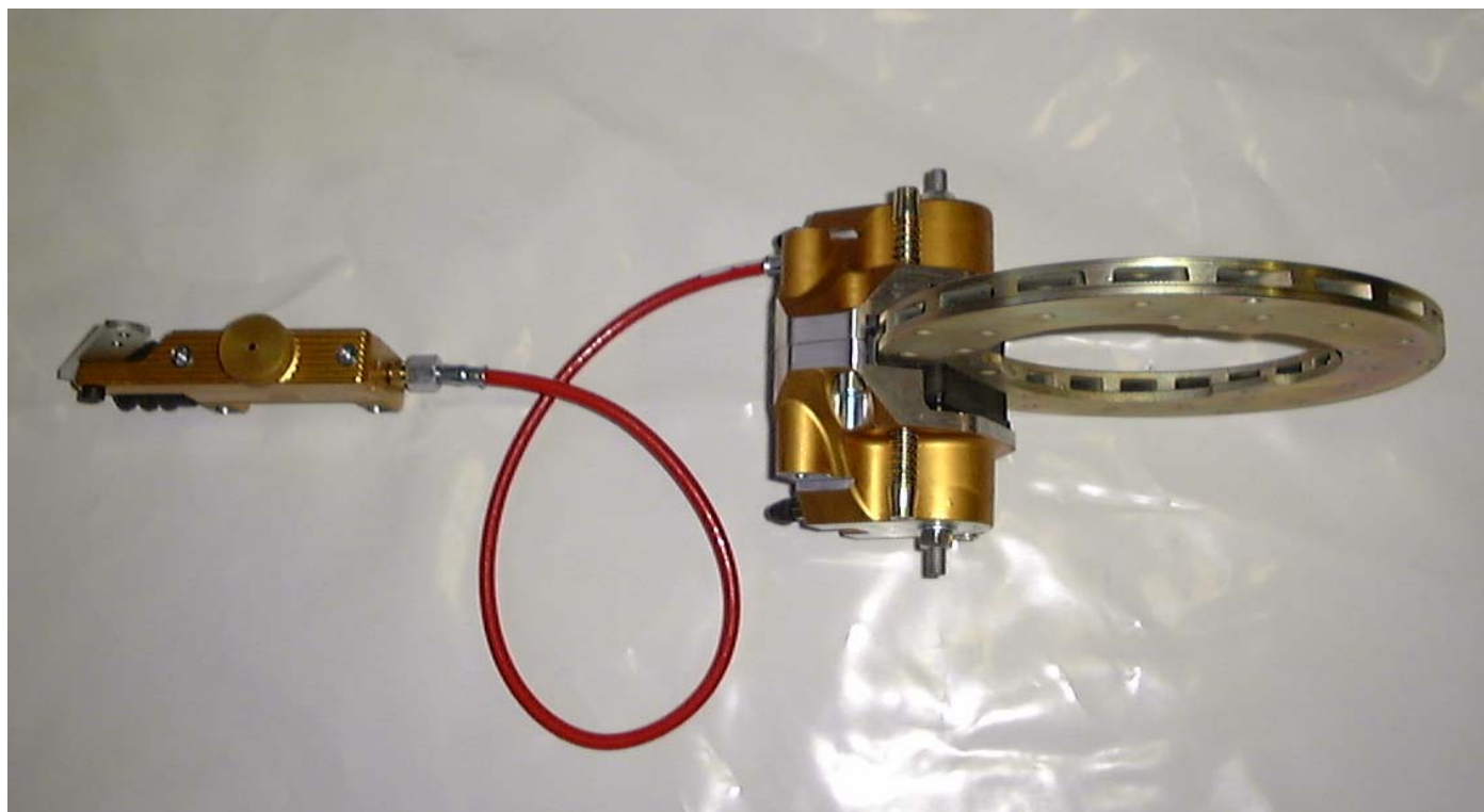
PHOTO VUE DE DESSUS DU SYSTÈME COMPLET
